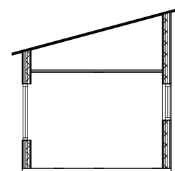
Sektion
